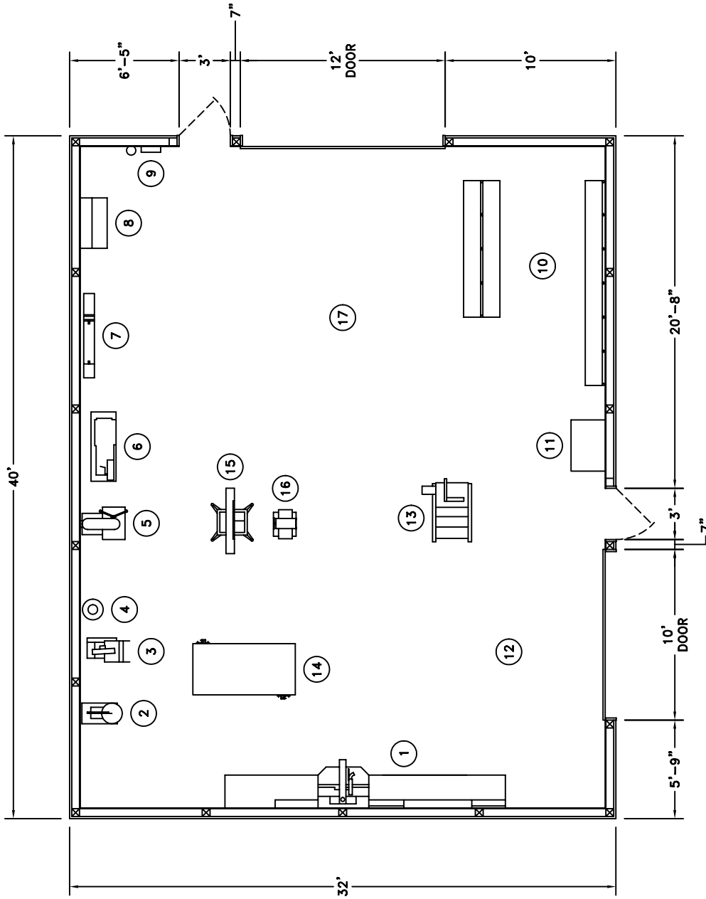
PLAN SCALE: 1/8"=1'-0"
